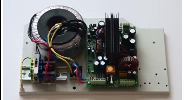
PZD13000/24V PLECH
