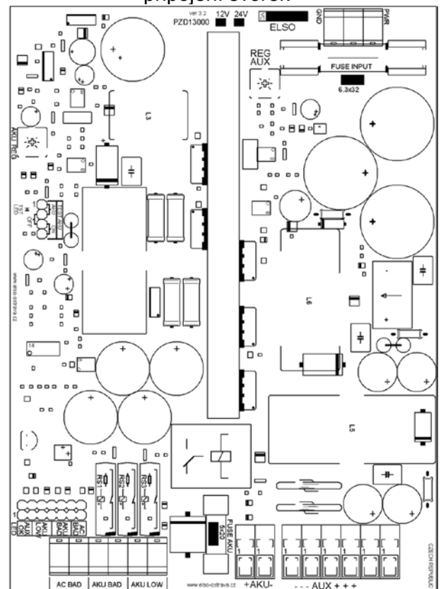
PZD130/24V připojení svorek
